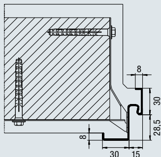
Profiel 11100
