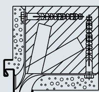
hoekkozijn Montage in metselwerk Muurplugankers
