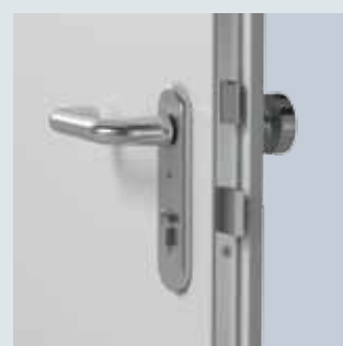
Uittrek- en doorboorbeveiligde veiligheid-wisselgarnituur
