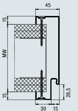
Profiel 21120 Spiegelschroefbevestiging
