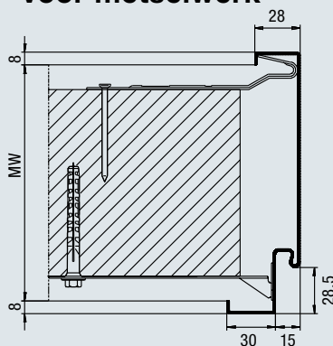
Profiel 21100
