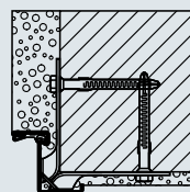
Montage met plugankers
