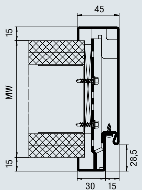
Profiel 21180 met opdek
