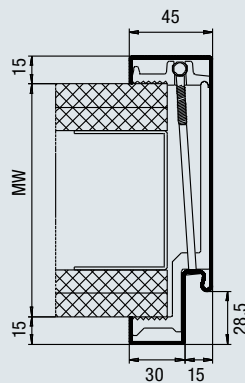
Profiel 21120 Klauwenbevestiging
