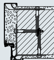
Hoekkozijn met aanvullend kozijn Montage met plugankers
