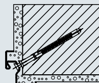
Speciaal hoekkozijn Plugmontage door de afdichtingsgroef
