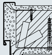
Muuromvattend kozijn Montage in metselwerk Muurplugankers
