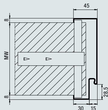
Profiel 21101
