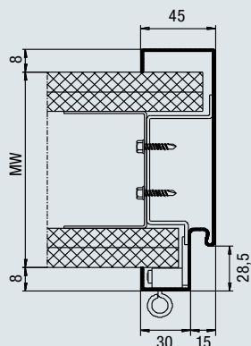
Profiel 21120
