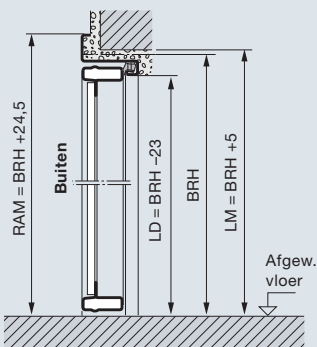
Buitenaanslag naar buiten openend
