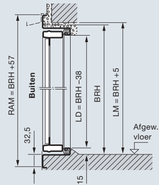
1-vleugelig met onderste aanslag
