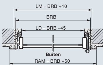
Buitenaanslag naar buiten openend
