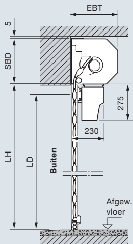
Maatbereik binnen- en buitenroldeur
