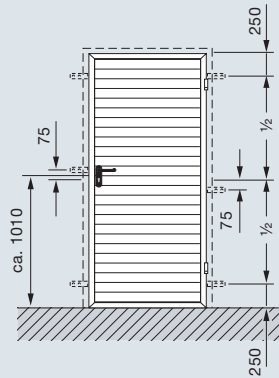
1-vleugelig zonder onderste aanslag
