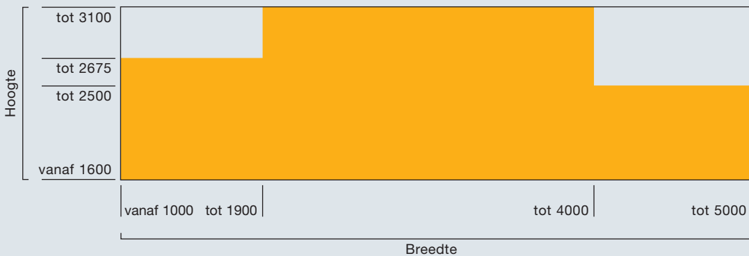
Maatbereik binnen- en buitenroldeur
