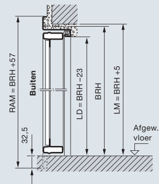
Binnenaanslag naar binnen openend
